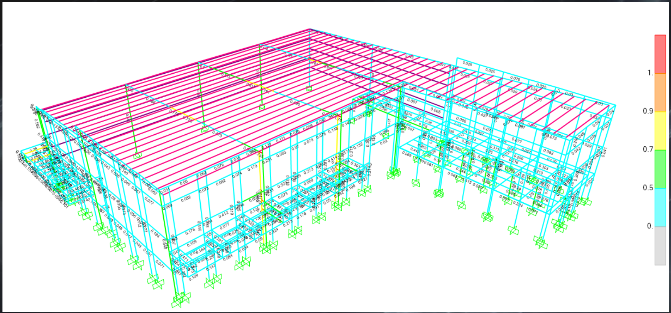
Calculo estructural nave
